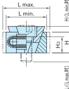
DK2-VT-F (平面)
