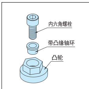
部件结构
