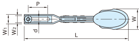
TCDHSL (带安全锁紧)
