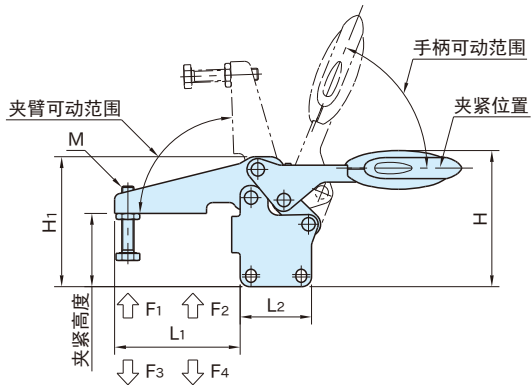
TCDHS (不带安全锁紧)
