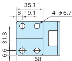
ST-PAH331 安装详细
