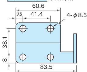
ST-PAH341 安装详细
