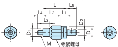
QLTL-RA (可卸型用接合器)
