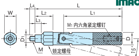
QLTL (标准型)
