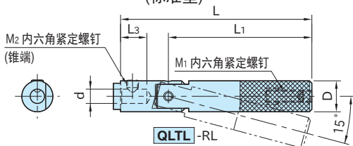
QLTL (标准型)
